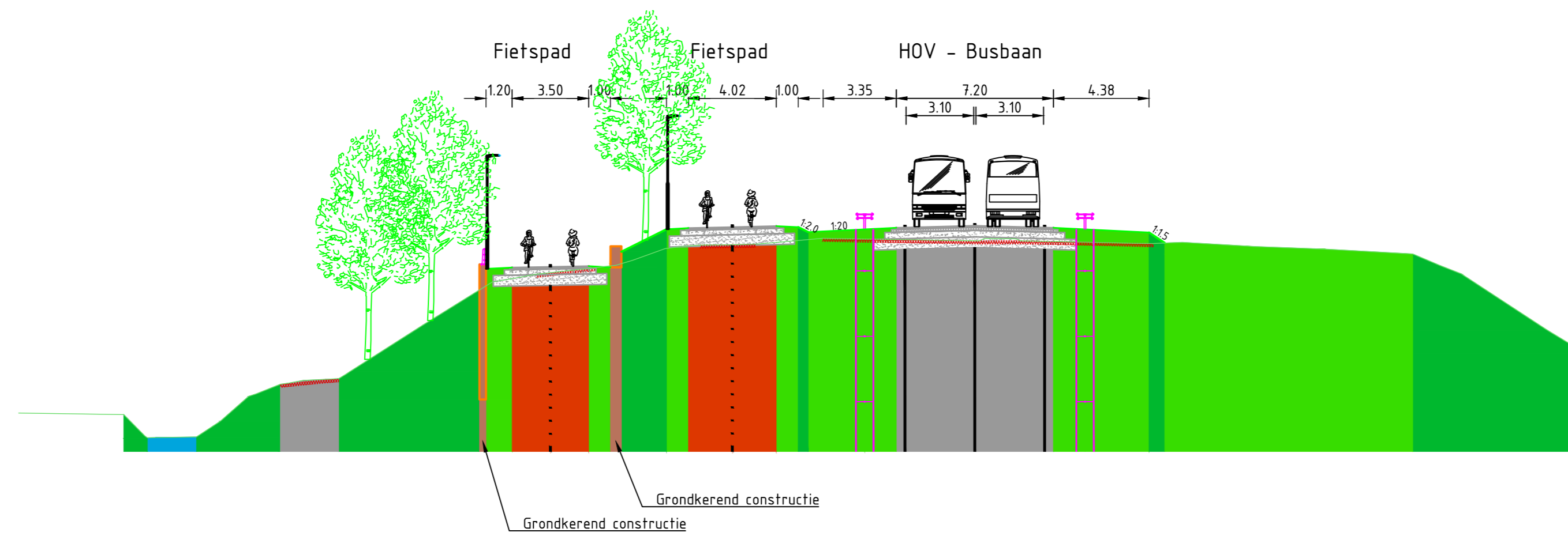
Dwarsprofiel ten zuiden van de Ringvaartbrug
