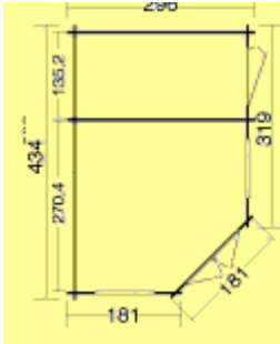
plattegrond tuinhuisje
